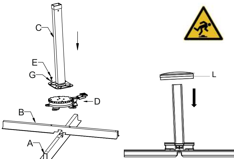
Abb. 3-1 Montage des Plattenständers
