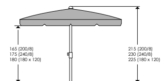
Abmessungen (cm):
