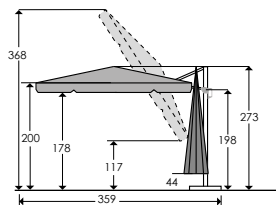
Abmessungen (cm)
