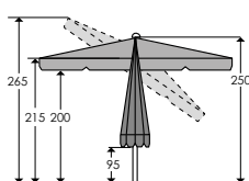
Abmessungen (cm):
