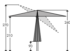
Abmessungen (cm):
